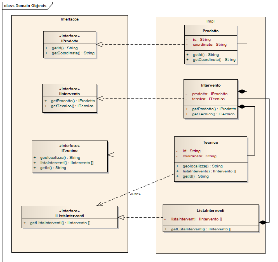
Figura 1.4: Modello del dominio
