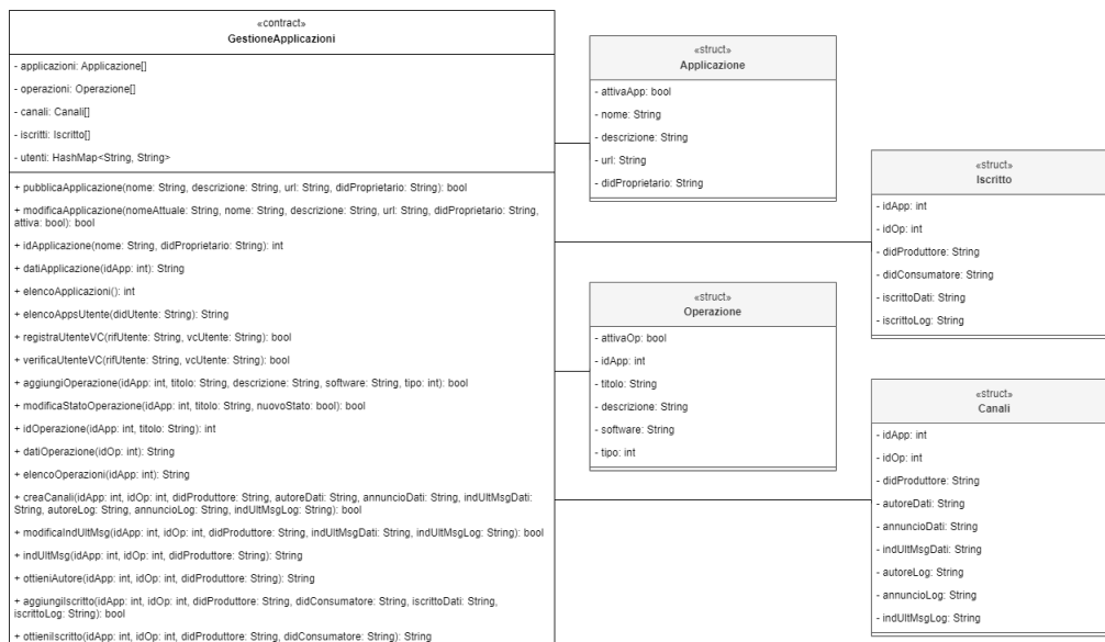
Figura 4.10: Diagramma UML dello smart contract GestioneApplicazioni
