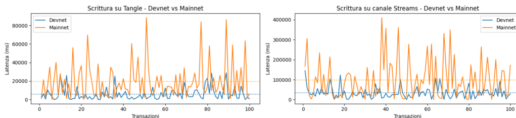
Figura 5.1: Grafici della latenza per le scritture sul Tangle e sui canali Streams
