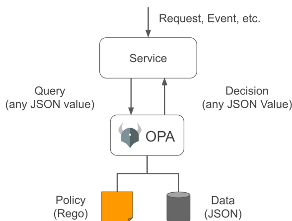
Figura 3.1: Meccanismo di operazione di OpenPolicyAgent . Si analizza la query proveniente da un servizio, e in base alle politiche e ai dati a sua disposizione, formula una decisione da inviare al mittente.
