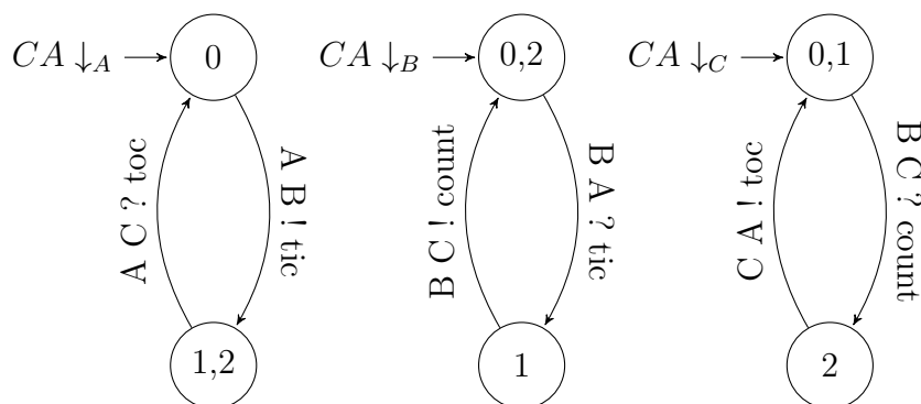
Figura 2.6: Le tre view locali estratte dall'automata in figura 2.5
