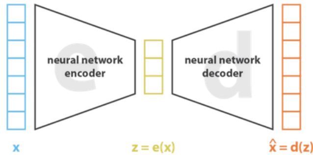
Figura 12: Struttura di un generico autoencoder [10].
