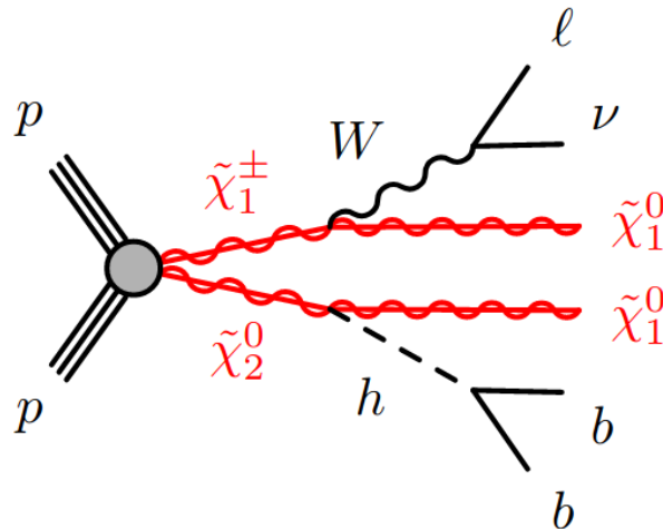
Figura 17: Diagramma del processo di produzione del chargino ( \tilde{\chi}_1^\pm ) e del neutralino pesante ( \tilde{\chi}_2^0 ).
