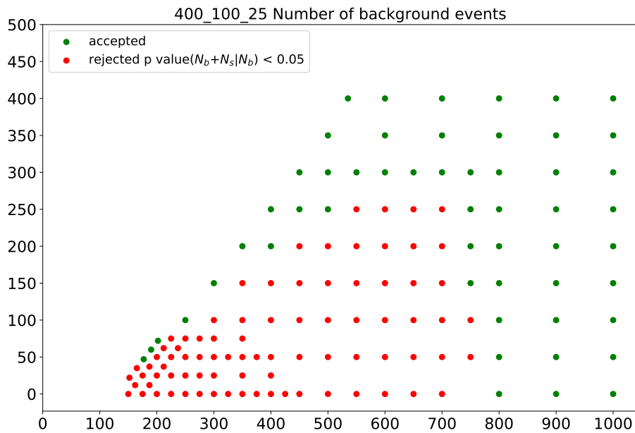
Figura 23: Risultato del processo di ottimizzazione nella distinzione fra fondo e segnale. Sono stati utilizzati i risultati ottimali in ciascuna delle tre zone individuate.
