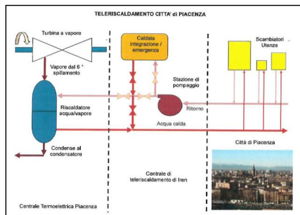
Figura 11: schema di funzionamento del teleriscaldamento Fonte: Emas 2009
