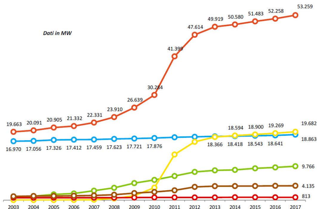
Figura 12: crescita della potenza ottenuta da risorse rinnovabili dal 2003 al 2017
