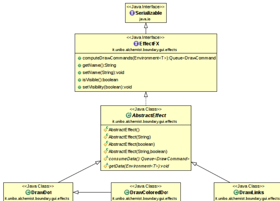
Figura 2.6: Diagramma UML delle classi che modellano la nuova struttura di effetti
