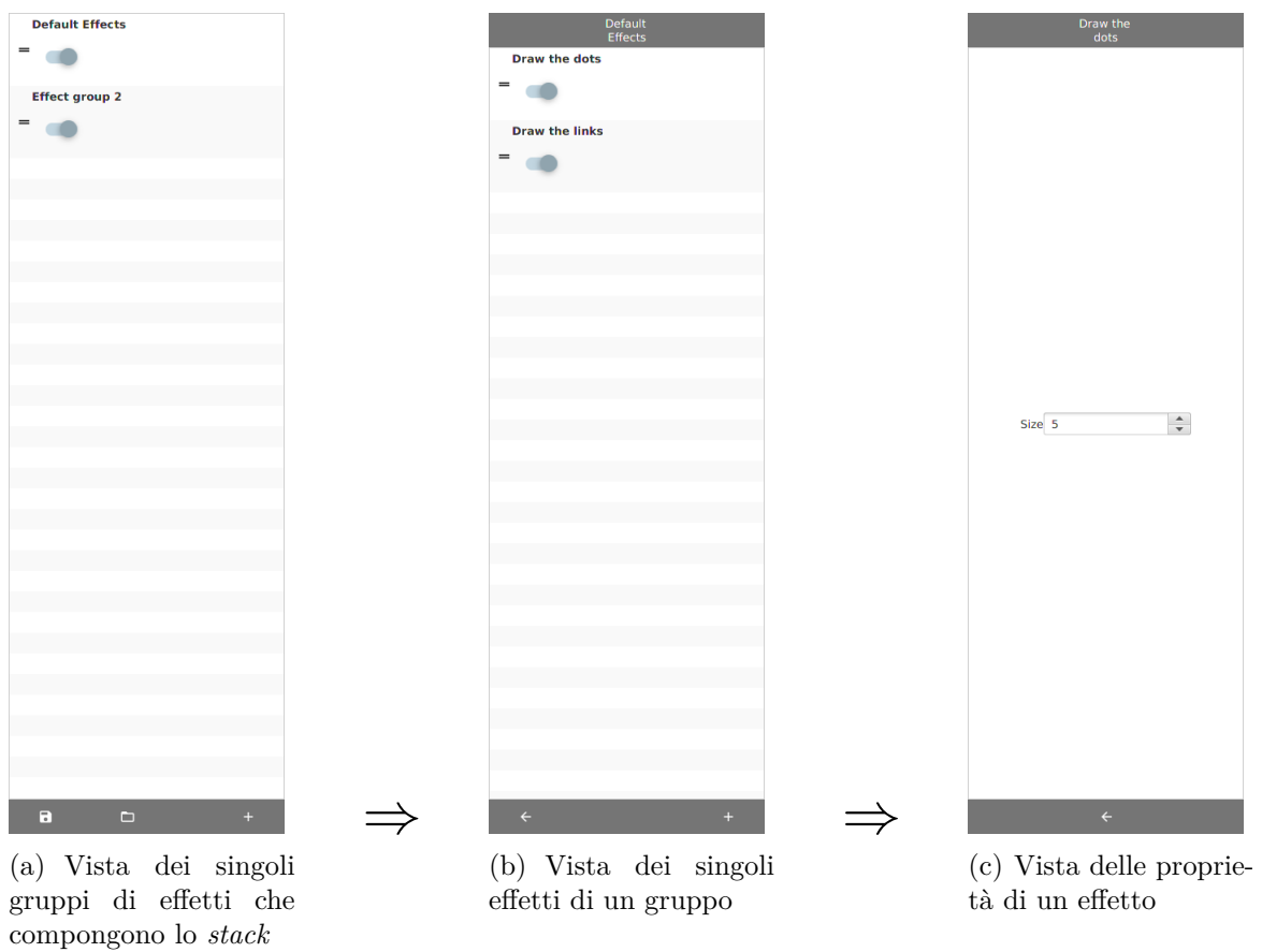
Figura 2.9: Vista del drawer laterale degli effetti nei diversi livelli
