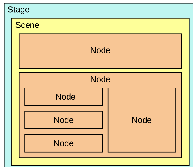
Figura 1.7: Struttura del layout di una applicazione JavaFX
