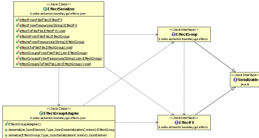
Figura 2.7: Diagramma UML delle classi che modellano la logica di serializzazione degli effetti tramite Facade stateless
