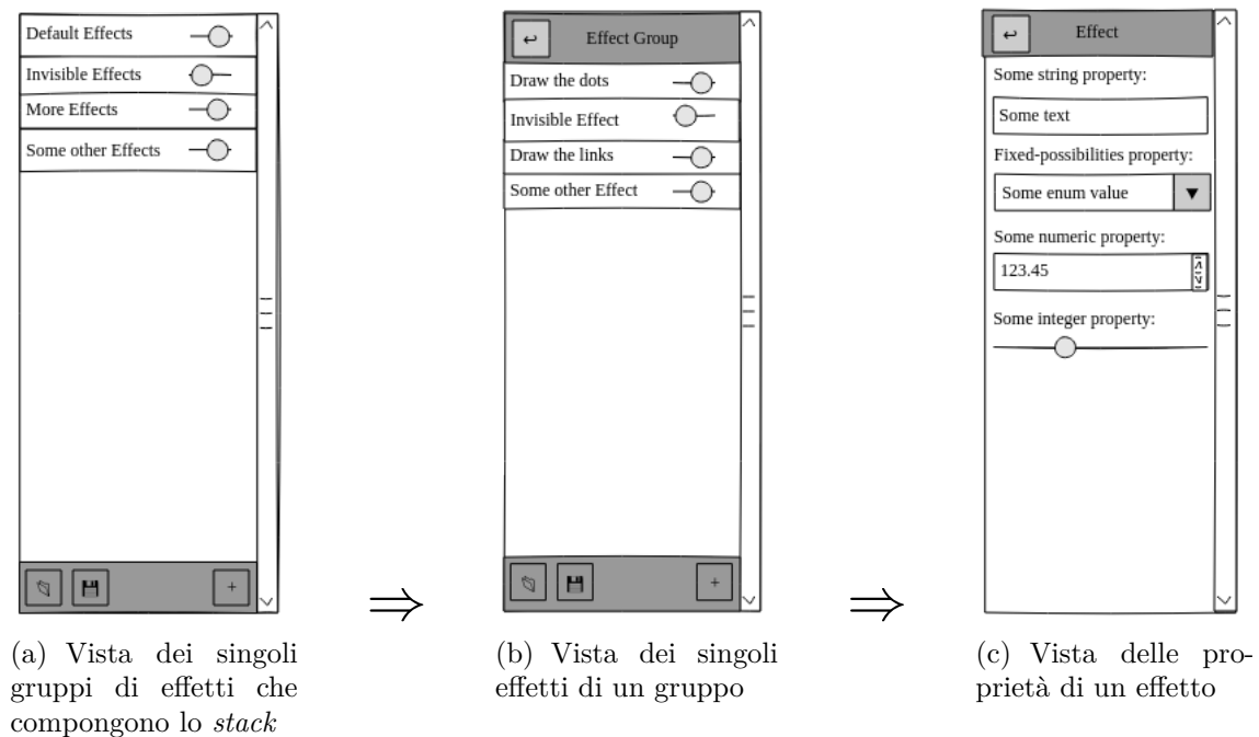
Figura 2.5: Mockup del pannello laterale degli effetti nei diversi livelli
