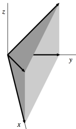
Figura 1.4: Cono poliedrale
