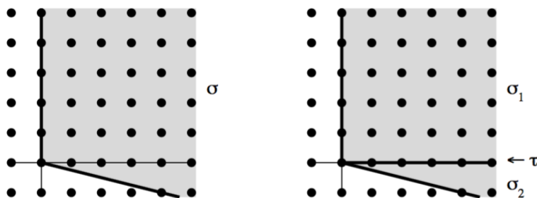
Figura 4.2: Il cono \sigma e il suo raffinamento dato da \sigma_1, \sigma_2, \tau
