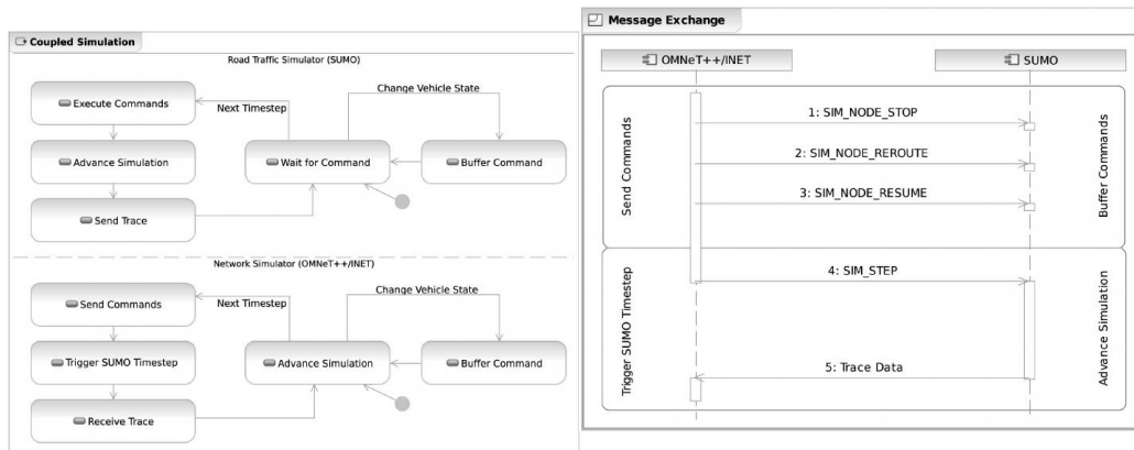
(a) Panoramica dei due simulatori abbinati. Macchina a stati di SUMO e i moduli di Veins. (b) Diagramma di sequenza dei messaggi scambiati tra SUMO e Veins. L'esecuzione dei comandi è ritardata fino al successivo passo temporale in SUMO.
