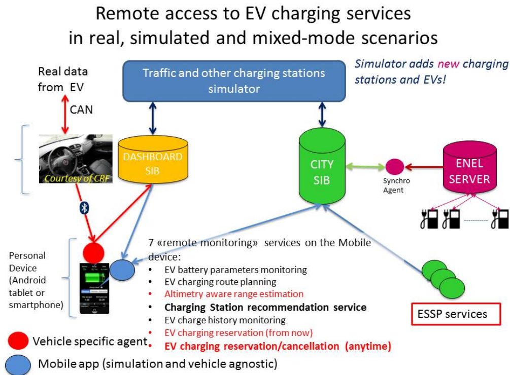
Figura 2.5: Architettura proposta per il progetto
