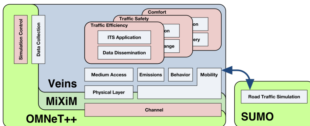
Figura 4.2: Architettura Veins
