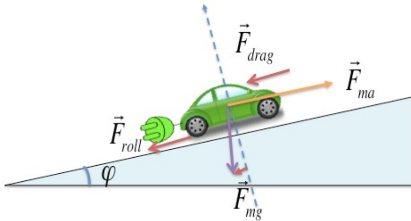
Figura 4.7: Schematizzazione del modello di consumo del veicolo
