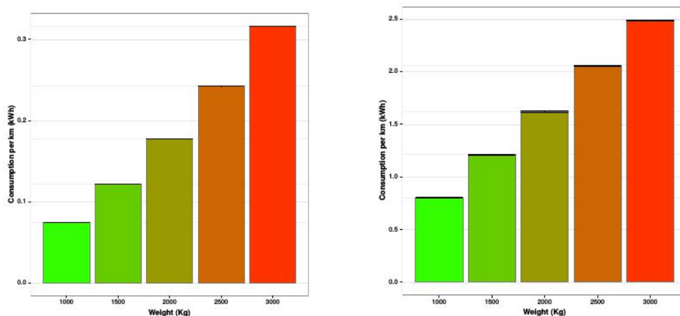
(a) Consumo del veicolo al variare del peso. Pendenza 0^\circ
