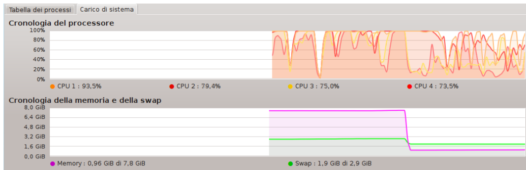
Figura 2.6: Memory Leak del SIB che avveniva quando la connessione viene interrotta da un socket-timeout
