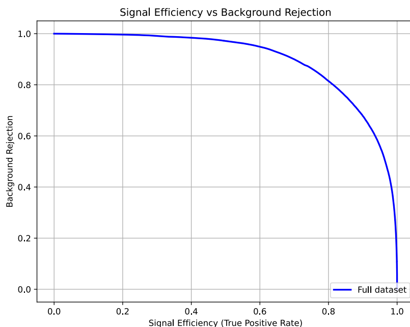
Figura 3.6: Curva di ROC dell'allenamento.
