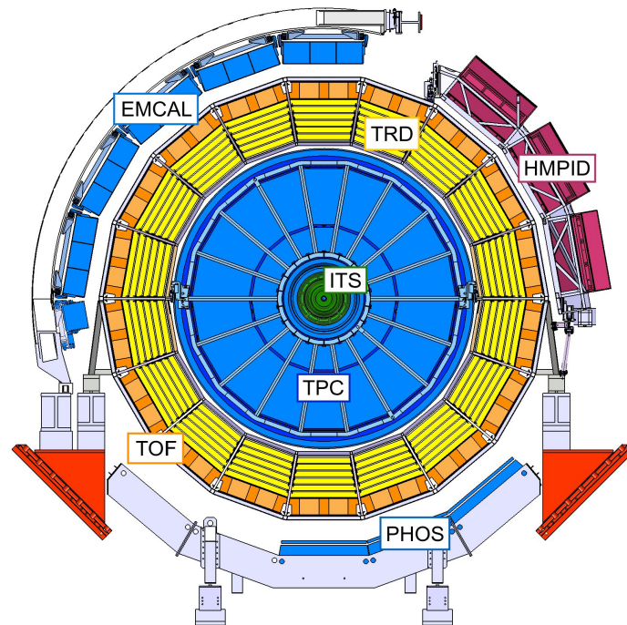
Figura 2.3: Sezione trasversale della parte centrale del rivelatore ALICE [44].
