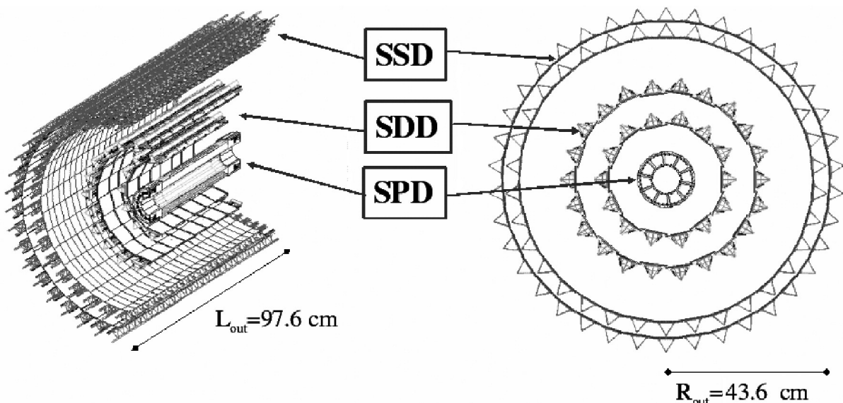
Figura 2.4: Spaccato e sezione interna dell'ITS di ALICE [17].
