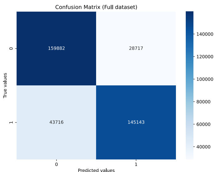
Figura 3.4: Confusion matrix dall'allenamento.
