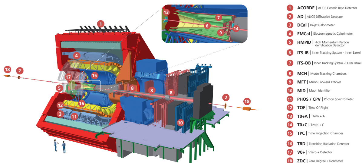
Figura 2.2: Spaccato del rivelatore ALICE con indicati i 18 sottorivelatori [43].
