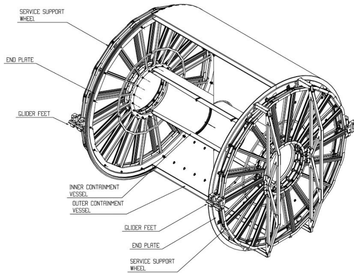
Figura 2.5: Rappresentazione schematica della struttura della TPC di ALICE [45].
