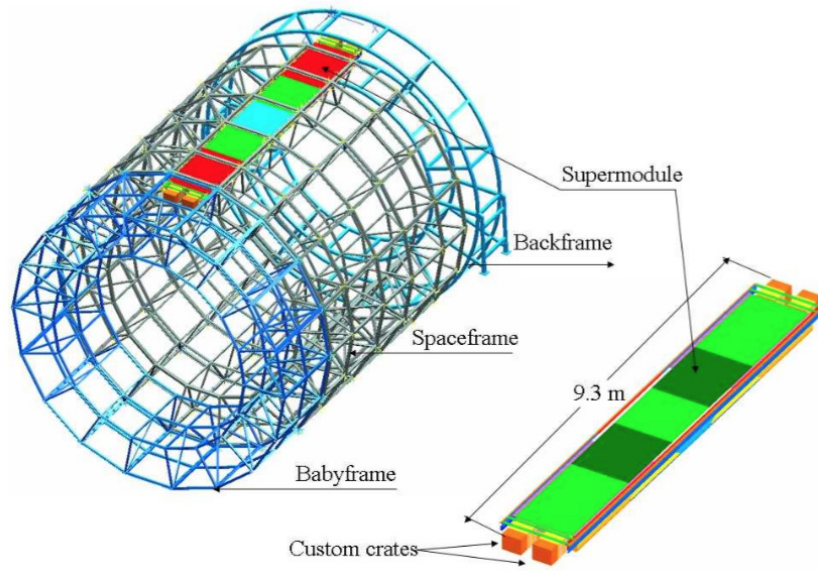
Figura 2.7: Rappresentazione schematica della struttura del TOF di ALICE [47].
