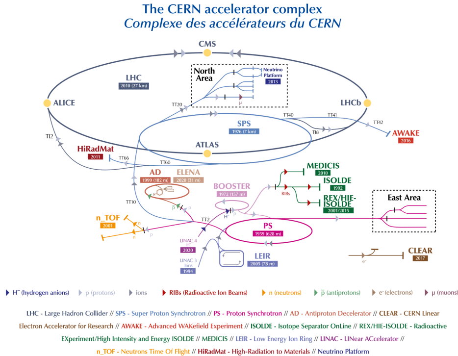
Figura 2.1: Sistema di rivelatori e acceleratori degli esperimenti del CERN di Ginevra [42].
