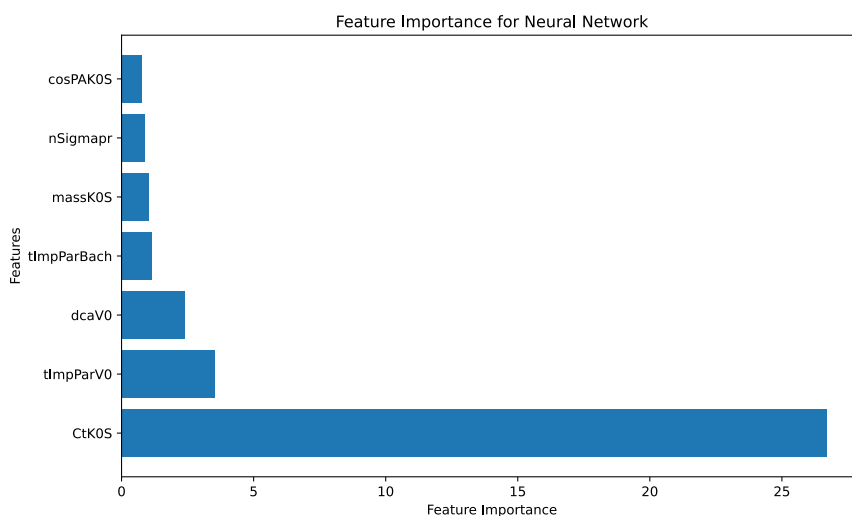
Figura 3.5: Ranking delle variabili di training.
