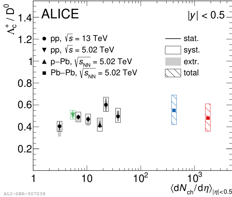
Figura 1.8: Valore del rapporto barione/mesone \Lambda_c^+/D^0 misurato dall'esperimento ALICE a LHC integrato su tutto lo spettro degli impulsi trasversi p_T del barione \Lambda_c^+ (sono stati utilizzati valori estrapolati dove non erano presenti misure sperimentali) per diversi sistemi collidenti: protone-protone pp, protone-nucleo p-Pb e nucleo-nucleo Pb-Pb, sia centrali sia periferici, in funzione della molteplicità [29]. Si può notare come il rapporto sia praticamente compatibile per tutti i tipi di collisioni entro gli errori sperimentali.
