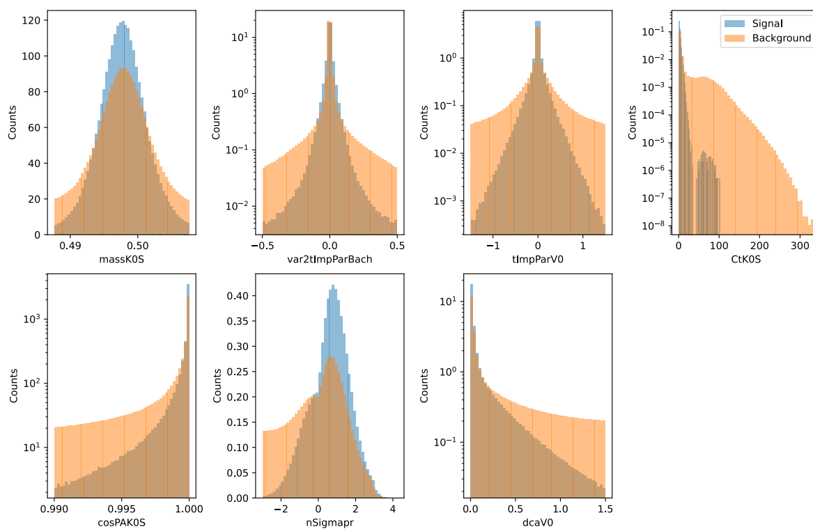
Figura 3.2: Variabili utilizzate per il classificazione degli eventi, viene messa in luce la differenza tra il segnale e il background.
