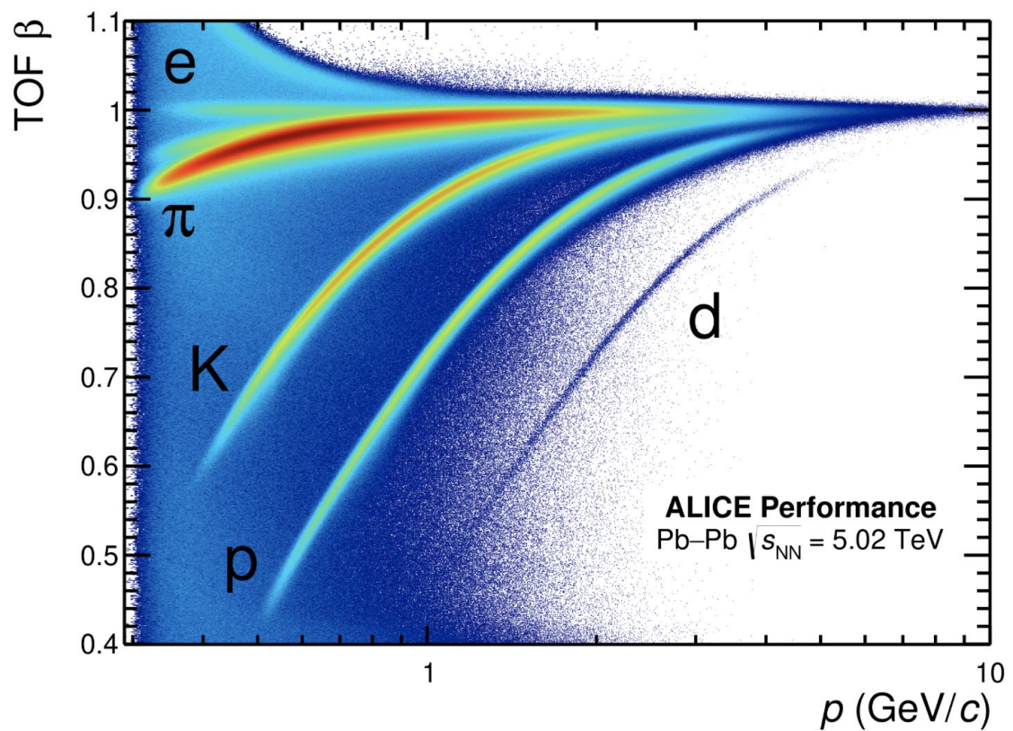
Figura 2.8: Velocità delle particelle cariche in funzione del loro impulso [48].
