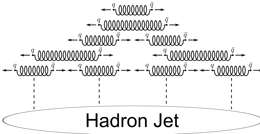
Figura 1.2: Rappresentazione grafica della rottura di stringa QCD nel vuoto [9]. La figura mostra come venga generata una coppia quark-antiquark quando un mesone riceve energia sufficiente: il gluone che lega i due quark si “allunga” finché non si spezza e forma una nuova coppia quark-antiquark.
