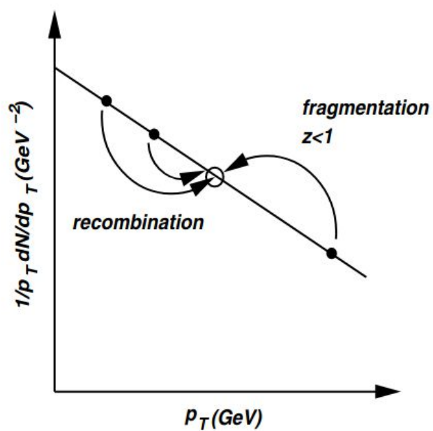
Figura 1.7: I meccanismi di ricombinazione e frammentazione in atto per creare lo stesso adrone nello stato finale in funzione dell'impulso trasverso p_T [28].
