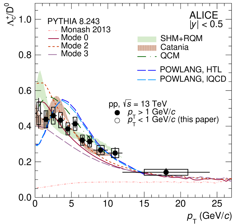
Figura 1.10: Rapporto di produzione \Lambda_c^+/D^0 in funzione dell'impulso trasverso p_T in collisioni pp a \sqrt{s} = 13 TeV confrontato con diversi modelli teorici [41].
