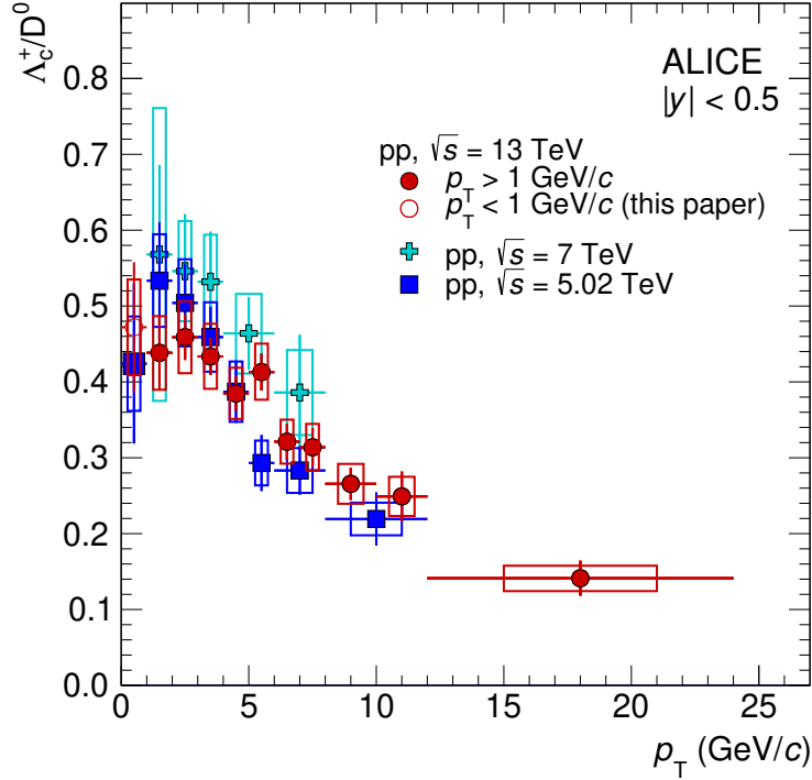
Figura 1.9: Rapporto di produzione degli adroni charmati \Lambda_c^+ e D^0 in funzione dell'impulso trasverso p_T in collisioni pp a energia cinetica nel centro di massa di \sqrt{s} = 5.02 TeV, \sqrt{s} = 7 TeV e \sqrt{s} = 13 TeV misurati col rivelatore ALICE a LHC [34].
