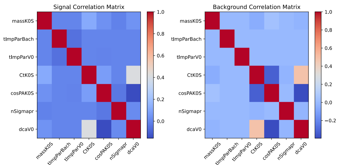
Figura 3.3: Matrici di correlazione lineare delle variabili in input a sinistra per il segnale e a destra per il fondo.
