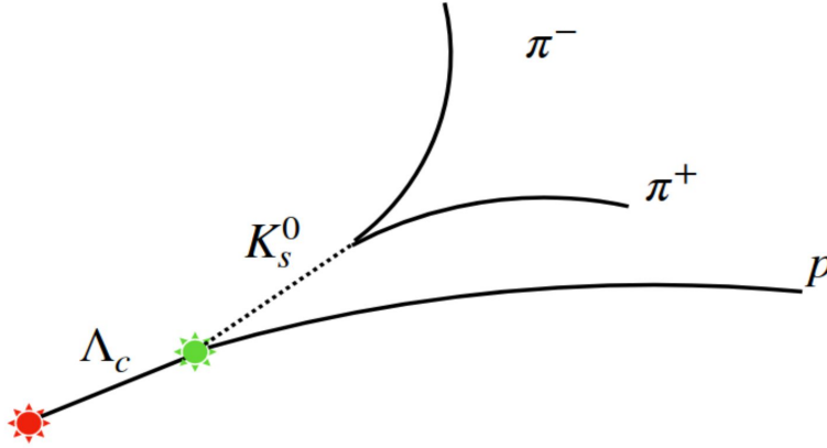
Figura 3.1: Rappresentazione grafica del decadimento del barione \Lambda_c^+ secondo il canale di decadimento 3.2 \Lambda_c^+ \rightarrow pK_s^0 [27].
