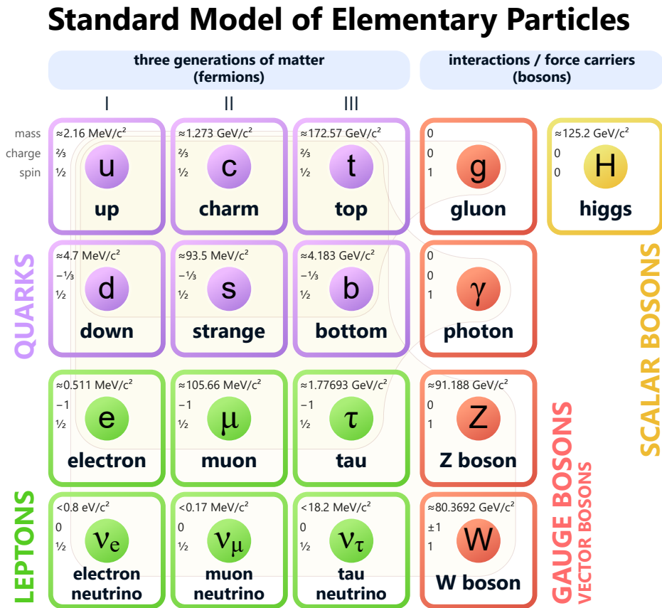
Figura 1.1: Schema delle particelle elementari presenti nel Modello Standard con relativa massa, carica e spin [2].
