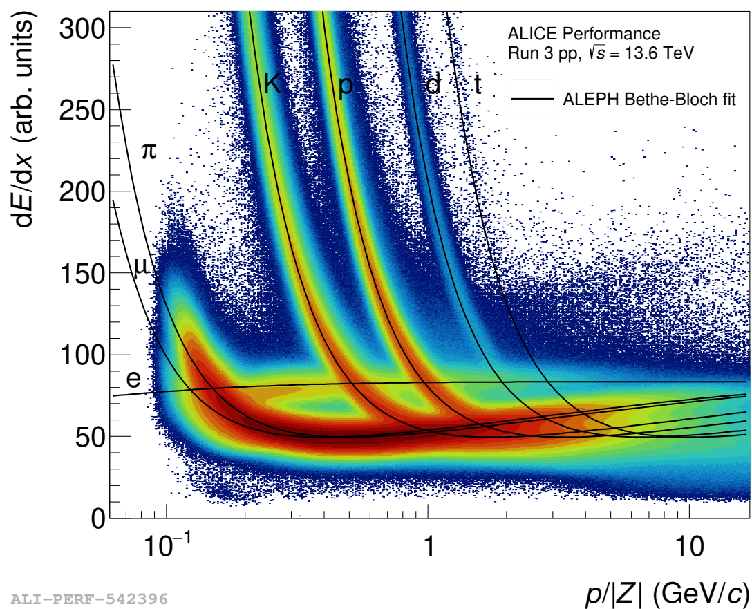
Figura 2.6: Misura della ionizzazione specifica in funzione dell'impulso della particella, è possibile notare come l'andamento vari in base al tipo di particella osservata [46].
