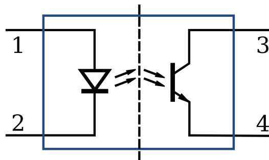
Figura 14: Un optoisolatore. Si può notare come questo contenga al suo interno un fototransistor (l'elemento sulla destra).
