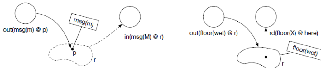
Figura 2.2: Agenti che inseriscono e recuperano tuple. A sinistra una out posiziona la tupla spaziale in una posizione specifica; una in recupera una tupla specificando una regione. A destra una out posiziona la tupla spaziale in una regione più grande; una rd osserva una tupla dalla posizione corrente [3].
