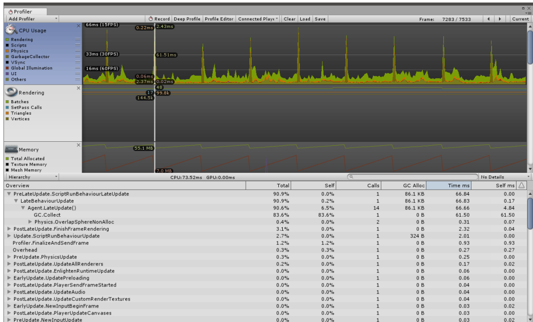
Figura 4.4: Profiler durante l'esecuzione del caso di studio Rescue con 14 agenti presenti nel MAS, su Android.
