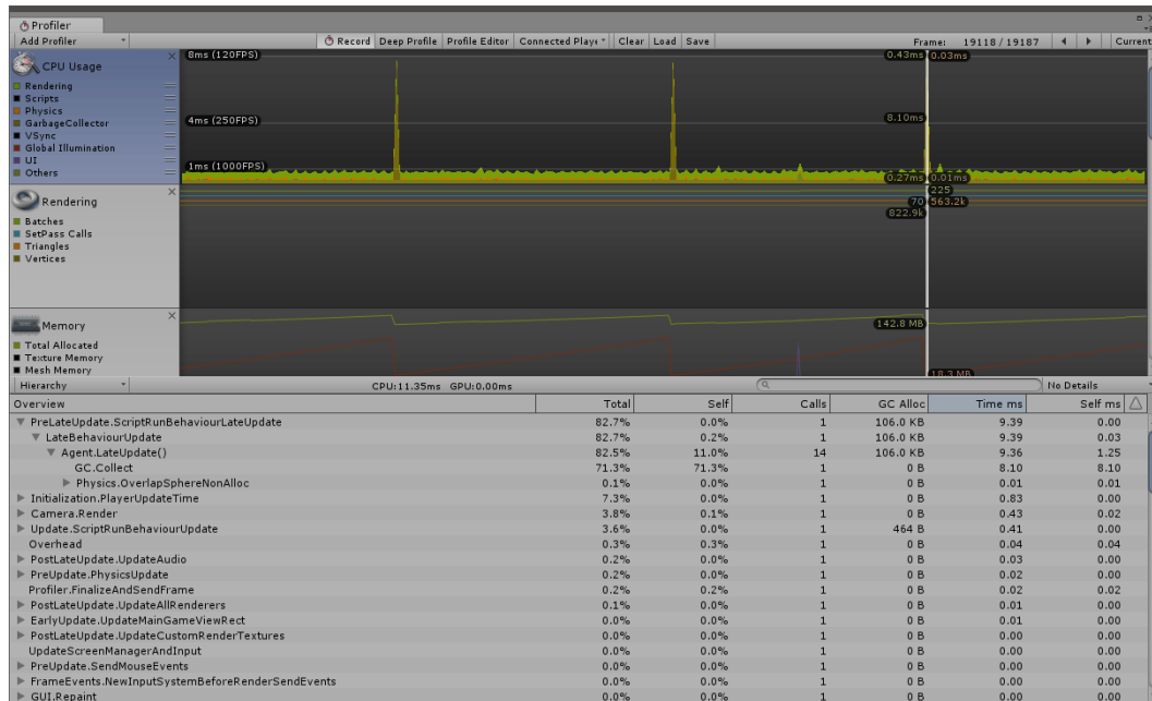
Figura 4.2: Profiler durante l'esecuzione del caso di studio Rescue con 14 agenti presenti nel MAS, su PC.
