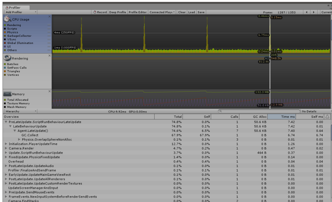
Figura 4.3: Profiler durante l'esecuzione del caso di studio Rescue con 7 agenti presenti nel MAS, su PC.
