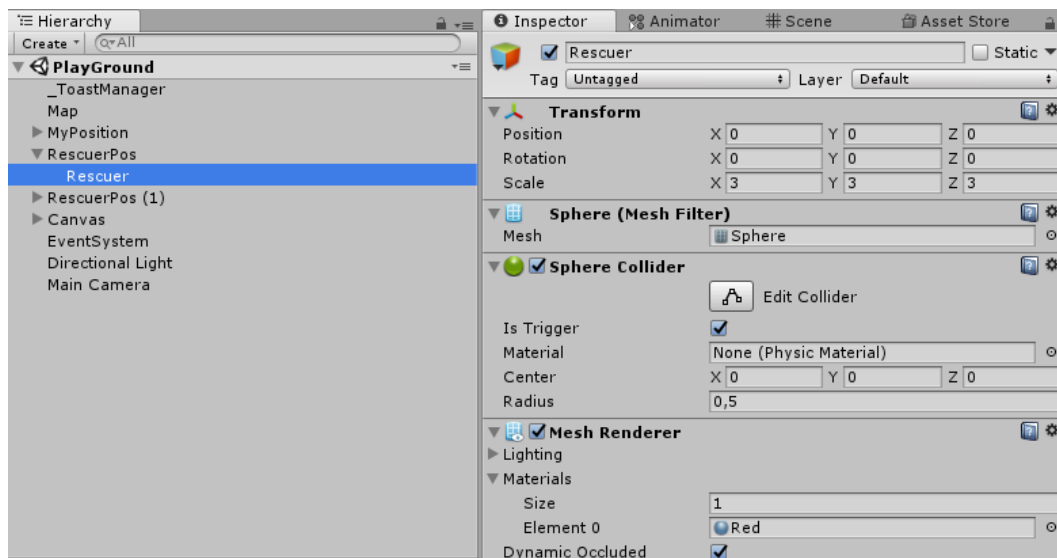
Figura 3.2: GameObject figlio a cui vengono applicati tutti i componenti Unity standard necessari
