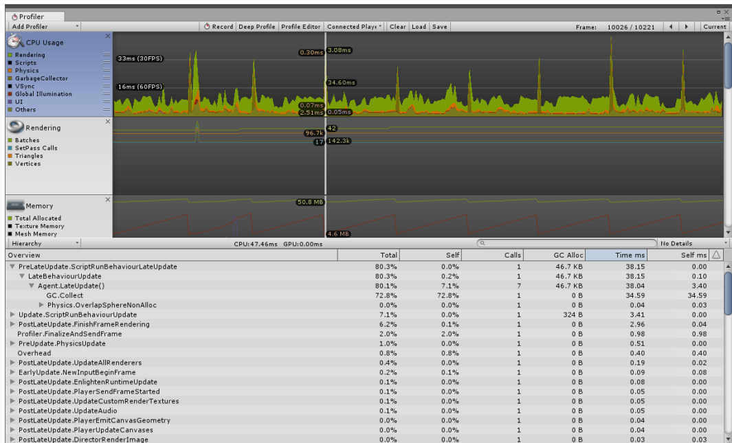
Figura 4.5: Profiler durante l'esecuzione del caso di studio Rescue con 7 agenti presenti nel MAS, su Android.
